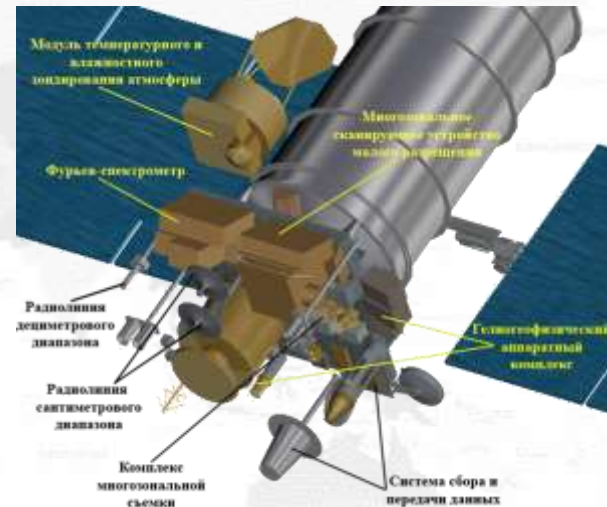
Основная целевая аппаратура космического аппарата «Метеор-М» №2-2
